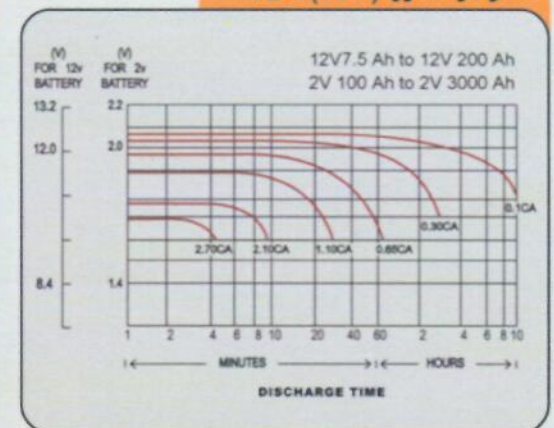
نمودار دشارژ ۲۵°C (۷۷°F)
