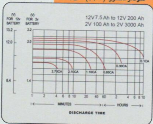
جدول میزان دشارژ و ولتاژ نهایی مطابق با استاندارد IEC60886-21
